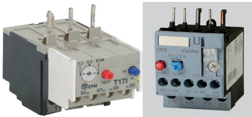
Obr. 8.5. Nadproudová relé, nahoře jsou patrné packy pro nasunutí do kontaktů stykače.
