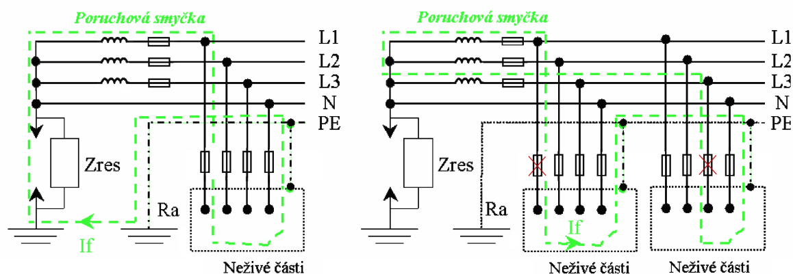
Obr. 6.10. Sít' IT – definice první a druhé poruchy a cesty poruchového proudu.
