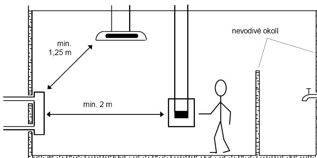
Obr. 7.3. Princip ochrany nevodivým okolím.
