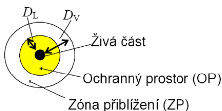
Obr. Vzdušné vzdálenosti a zóny pro pracovní postupy
