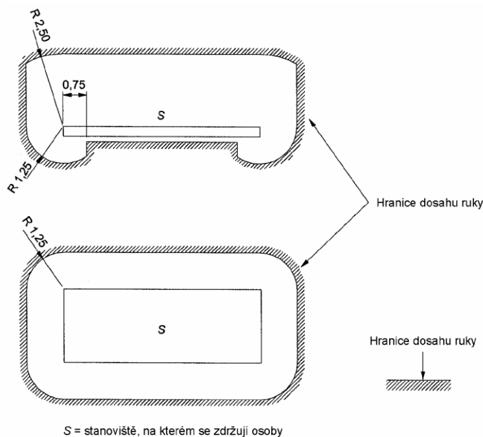
Obr. 7.1. Ochrana polohou, hranice dosahu ruky.
