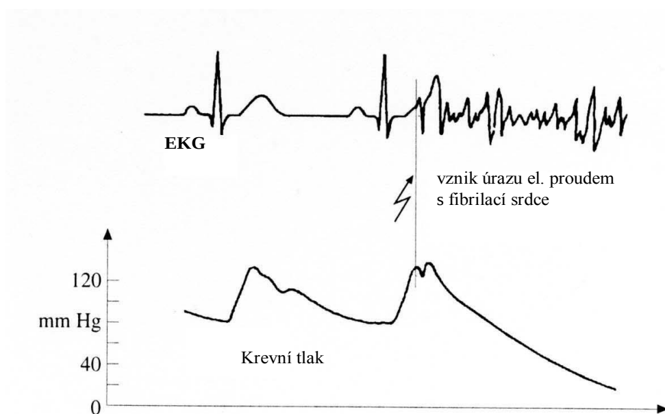
Obr. 12.1 Průběh EKG a krevního tlaku před a po vzniku úrazu elektrickým proudem
